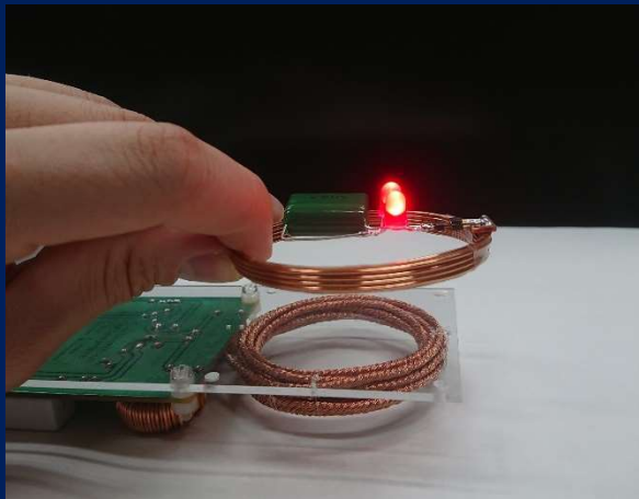
<無線給電により空中で光る発光ダイオード>
